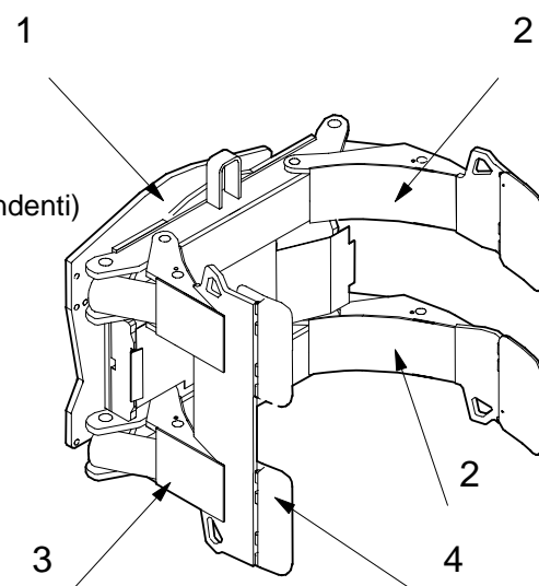
Figura: Componenti principali della pinza della serie RA
