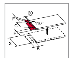
Überfahrblech
