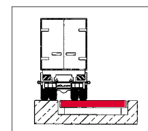
Plattformverstärkung LKW-überfahrbar
