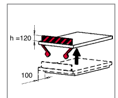
Placa de contención por contrapeso
