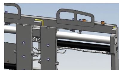
Beidseitiger Schutz der Anschlußhydraulik (nur Typen 06/09/10/12)
